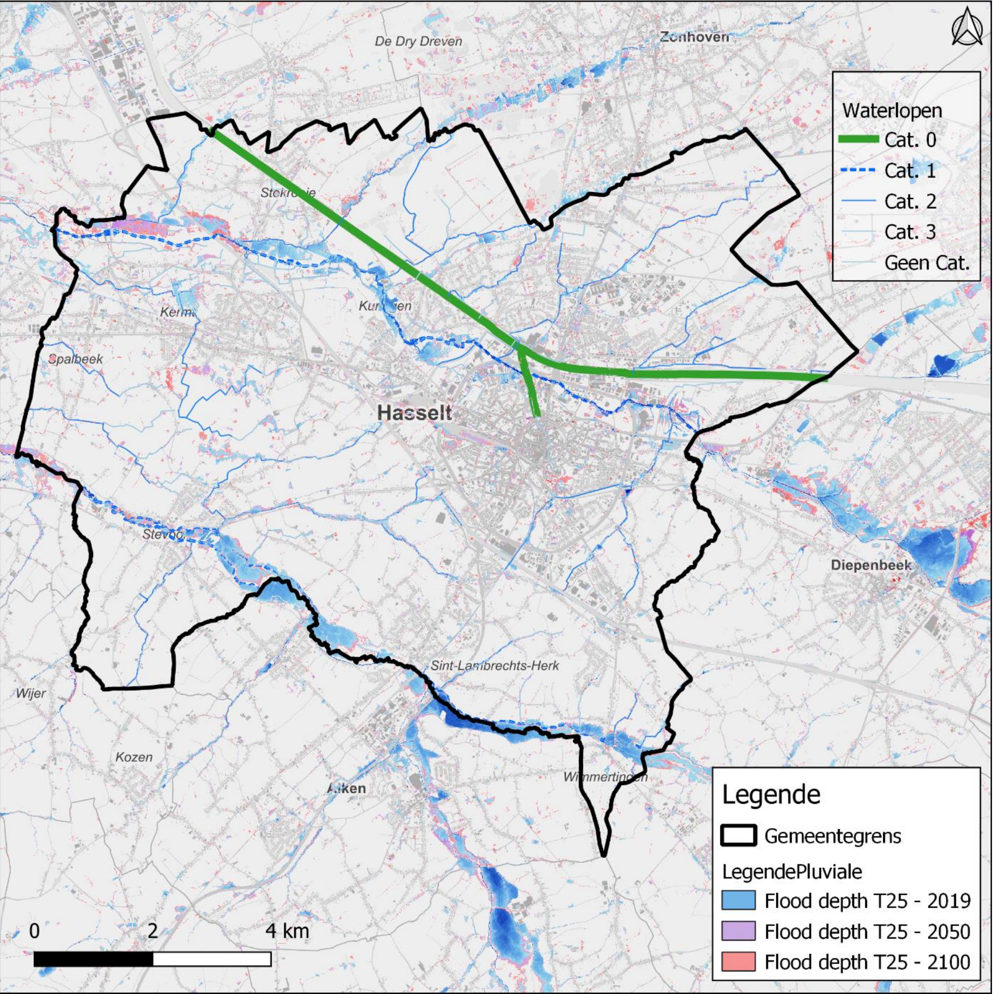
Pluviale overstromingskaart Stad Hasselt
